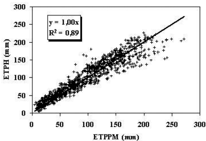
FIGURA 1 – Relação entre os valores mensais da evapotranspiração potencial calculados pelos métodos de Penman-Monteith (ETPPM) e de Hargreaves (ETPH).
