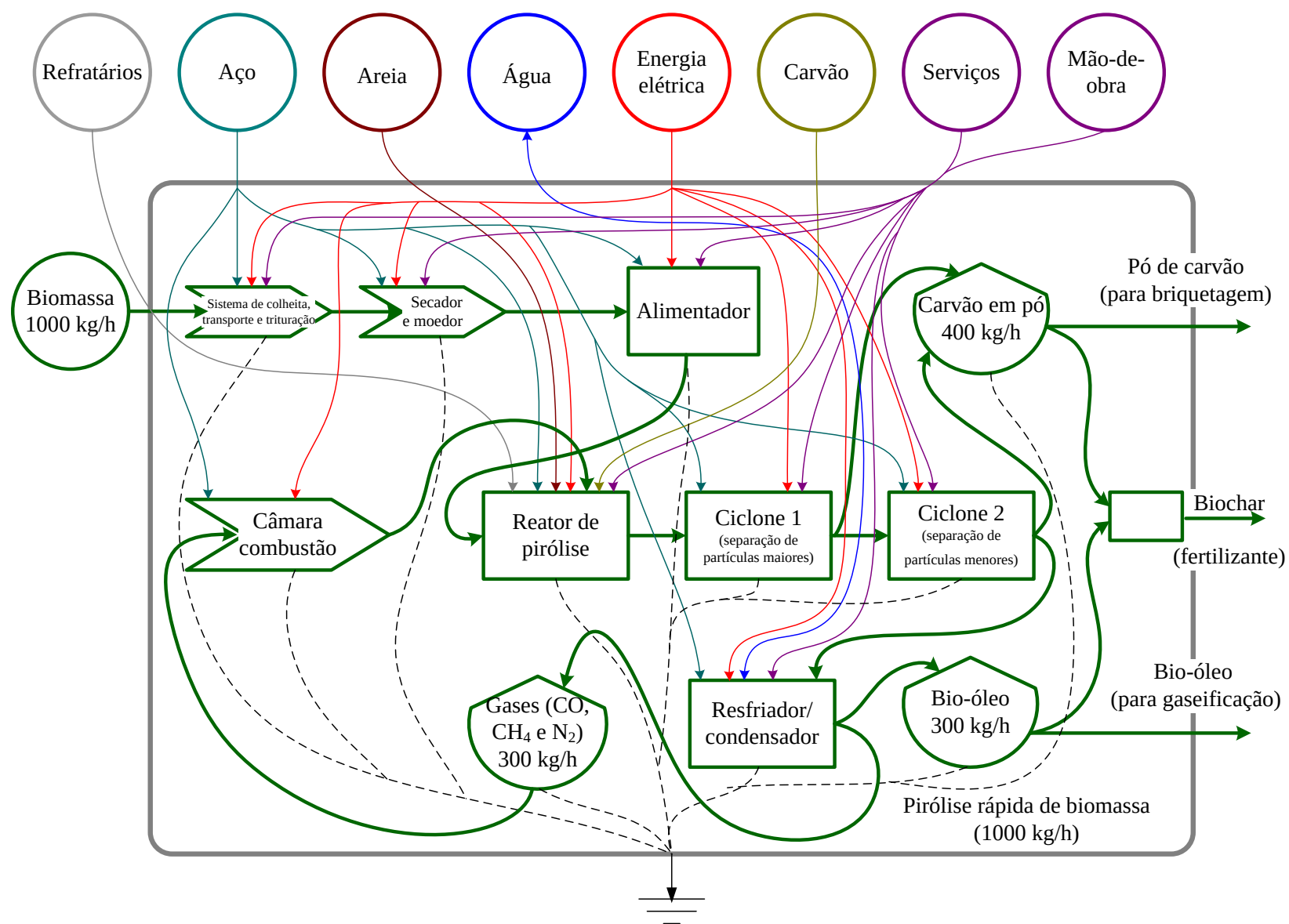
Figura 25. Diagrama detalhado do processo de pirólise rápida de biomassa para obtenção de bio-óleo e bio-carvão
