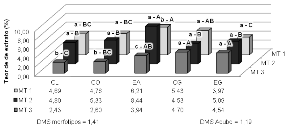
Figura 10: Teor de extrato (%) em folhas de três morfotipos de A. chica : morfotipo 1 (MT1); morfotipo 2 (MT2) e morfotipo 3 (MT3), cultivadas sob condições de campo, em função das fontes de adubo orgânico: controle (CL); composto orgânico (CO); esterco de aves (EA); casca de guaraná (CG) e esterco de gado (EG) em Manaus, AM. 2010-11. Médias seguidas de mesma letra na coluna (minúscula) comparam entre si os morfotipos enquanto as letras na linha (maiúsculas) comparam entre si os adubos, não diferindo entre si pelo Teste de Tukey ( p < 0,05 ).
