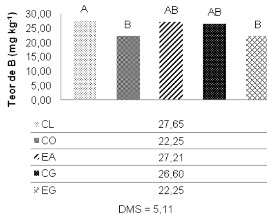
Figura 15: Teor médio de boro (B) em folhas de três morfotipos de A. chica : morfotipo 1 (MT1); morfotipo 2 (MT2) e morfotipo 3 (MT3), cultivadas sob condições de campo, em função das fontes de adubo orgânico: controle (CL); composto orgânico (CO); esterco de aves (EA); casca de guaraná (CG) e esterco de gado (EG) em Manaus, AM. 2010-11. Médias seguidas pela mesma letra não diferem entre si pelo Teste de Tukey ( p < 0,05 ).
