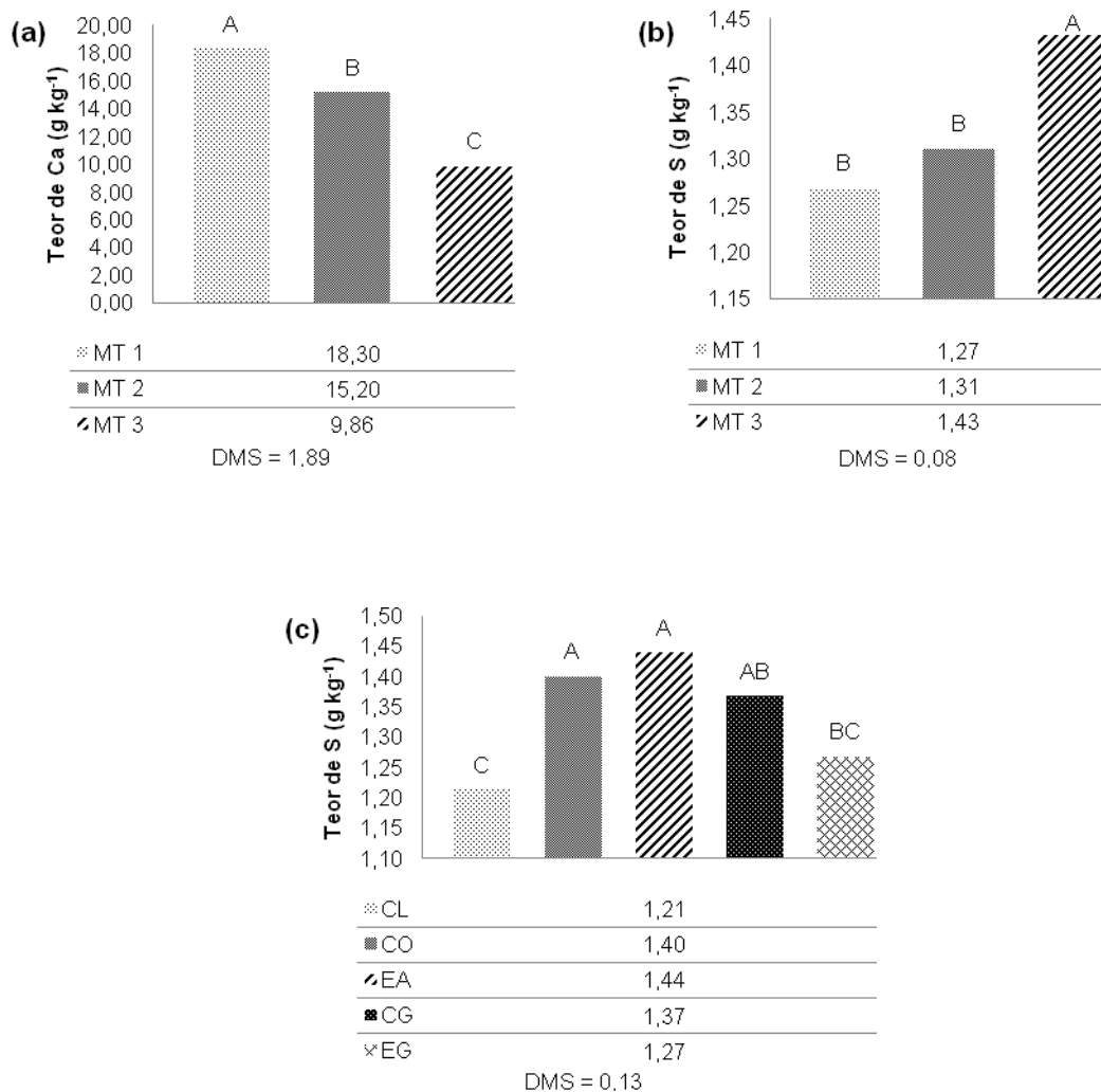
Figura 14: Teores médios de cálcio (a), enxofre (b e c) em folhas de três morfotipos de A. chica : morfotipo 1 (MT1); morfotipo 2 (MT2) e morfotipo 3 (MT3), cultivadas sob condições de campo, em função das fontes de adubo orgânico: controle (CL); composto orgânico (CO); esterco de aves (EA); casca de guaraná (CG) e esterco de gado (EG) em Manaus, AM. 2010-11. Médias seguidas pela mesma letra não diferem entre si pelo Teste de Tukey ( p < 0,05 ).
