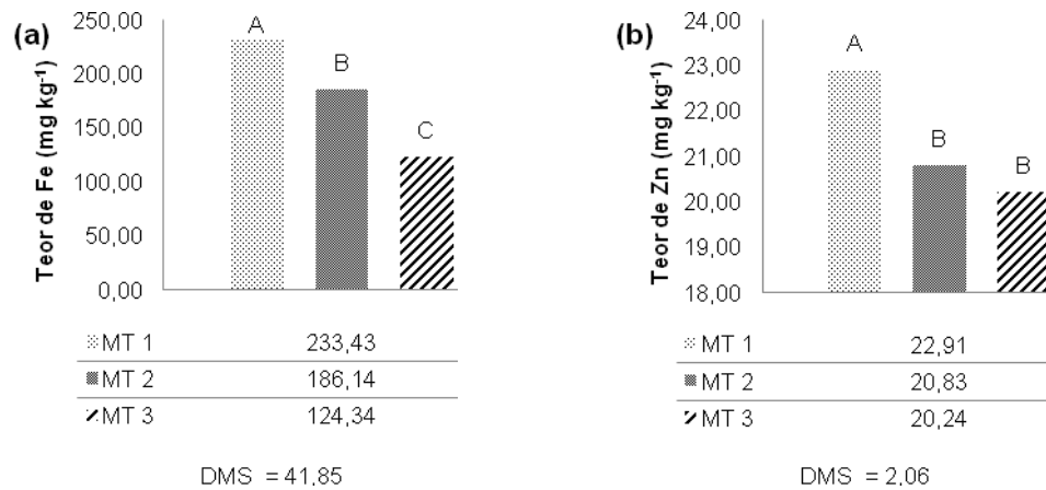
Figura 17: Teor médio de ferro (Fe) (a) e Zinco (Zn) (b) em folhas de três morfotipos de A. chica : morfotipo 1 (MT1); morfotipo 2 (MT2) e morfotipo 3 (MT3), cultivadas sob condições de campo, em função das fontes de adubo orgânico: controle (CL); composto orgânico (CO); esterco de aves (EA); casca de guaraná (CG) e esterco de gado (EG) em Manaus, AM. 2010-11. Médias seguidas pela mesma letra não diferem entre si pelo Teste de Tukey ( p < 0,05 ).
