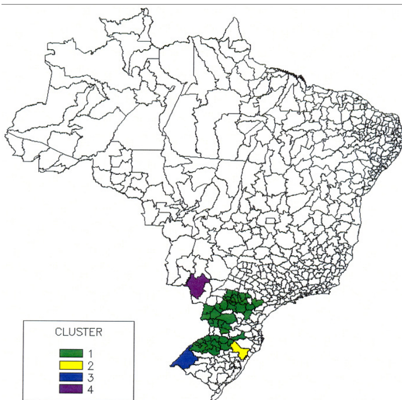
Figura 1: Clusters com grande participação na produção de trigo no Brasil
