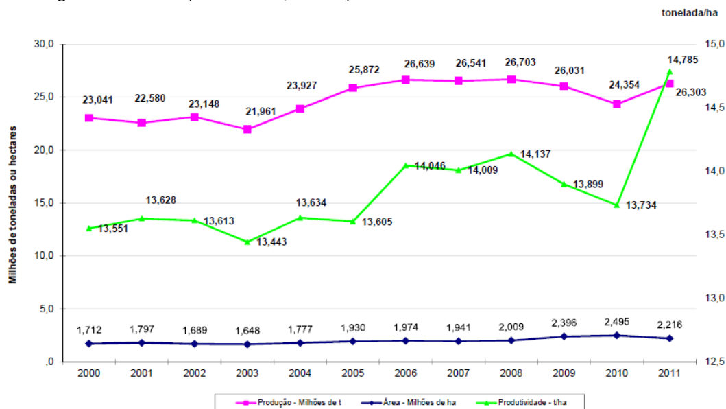
Figura 12 – Evolução da Área, Produção e Produtividade da Mandioca no Brasil
