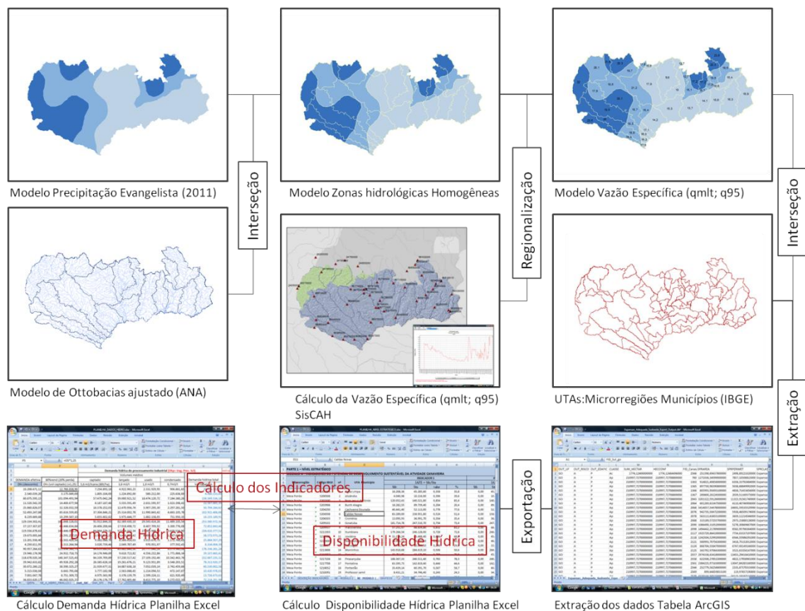
Figura 36 - Apresentação esquemática da metodologia para a elaboração modelo de vazão específica, extração e cálculo dos indicadores de sustentabilidade hídrica (ICDHs, IAMEs, ICDHi, IAMEi).
