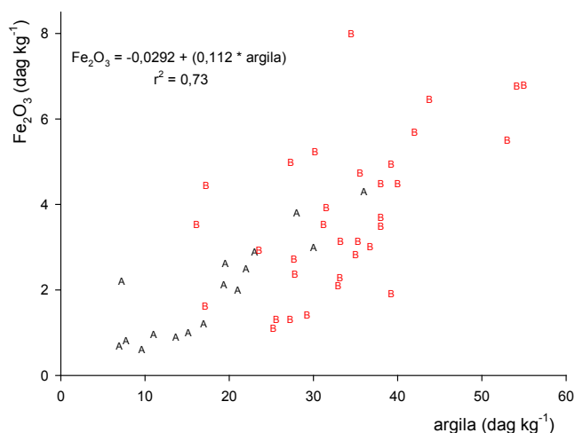
Figura 6. Teores de \text{Fe}_2\text{O}_3 do ataque sulfúrico em função da argila. Legenda: A – amostras do horizonte A; B – amostras do horizonte B. N = 49.
