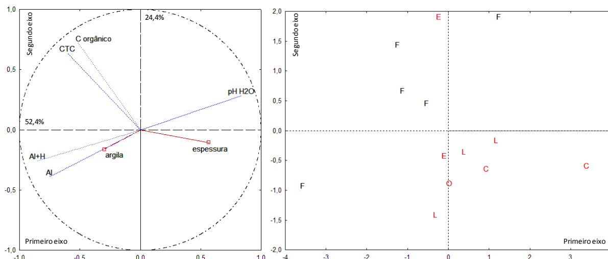
Figura 7. Análise de componentes principais de amostras superficiais dos solos estudados e agrupados pelo uso atual. (A) Círculo de autovetores das variáveis (CTC = capacidade de troca catiônica), sendo vetores em vermelho de variáveis suplementares, e autovalores dos eixos; (B) Plano de dispersão de pontos. Códigos de cada grupo: F = floresta, C = cana-de-açúcar; L = laranja; O = coco; E = eucalipto (usos da terra diferentes de floresta, em vermelho).
