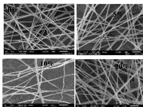
Fig. 2. Nanofibras de PHBV + Diclofenaco de sódio obtidas por fiação por sopro.
