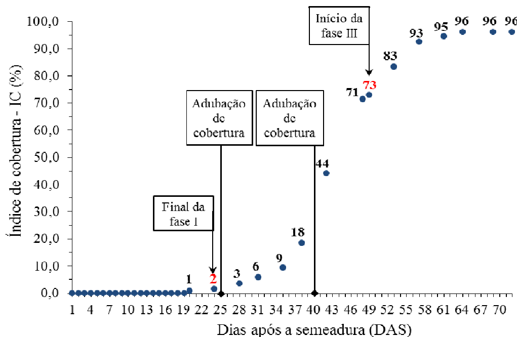
Figura 2. Evolução do índice de cobertura do solo pela vegetação (IC), valores médios entre os IC da área interna e externa aos lisímetros, durante o ciclo da cultura da melancieira e detalhes dos valores do IC no final da fase I e início da fase III e dos dias de adubação de cobertura.
