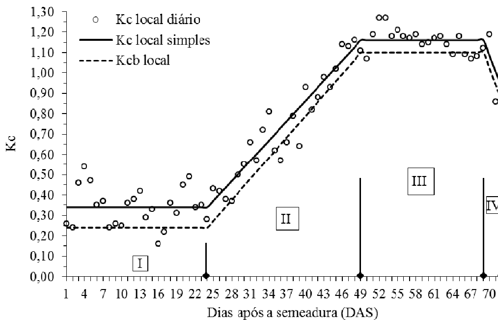
Figura3. Variação diária do coeficiente de cultura ( K_c local diário) e curvas de K_c simples ( K_c local simples) e de K_c basal ( K_{cb} local) em função das fases da cultura da melancia.
