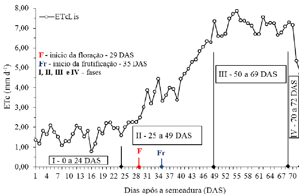
Figura 1. Evapotranspiração diária da cultura de melancia medida com os lisímetros (ETcLis) e divisão do ciclo da cultura em fases de acordo com o comportamento da curva de ETc.
