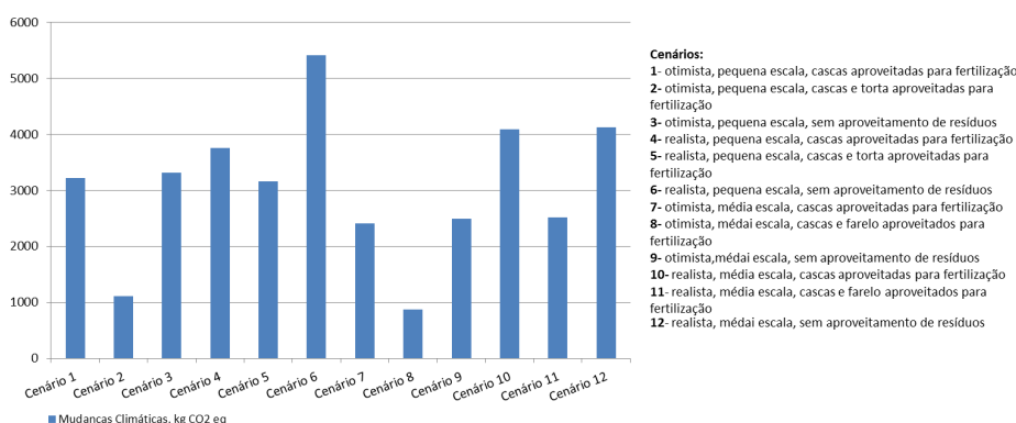
Figura 3. Mudanças Climáticas.
