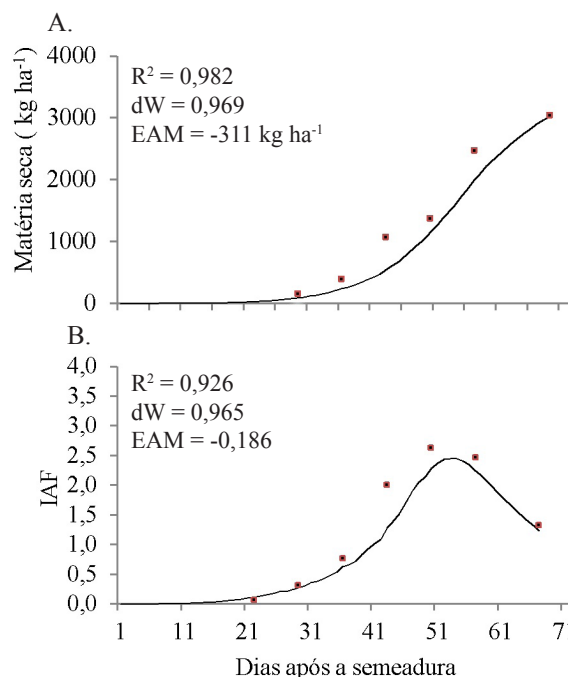
Figura 2. Estimativa de matéria seca em (A) e de índice de área foliar (IAF) em (B) na fase de calibração
