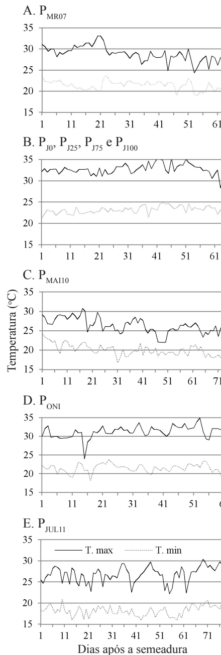
Figura 5. Valores das temperaturas máxima e mínima ocorridas durante os cultivos P MAR07 (A), de janeiro de 2010 (B), P MAI10 (C), P ONI (D) e P JUL11 (E) em Cruz das Almas
