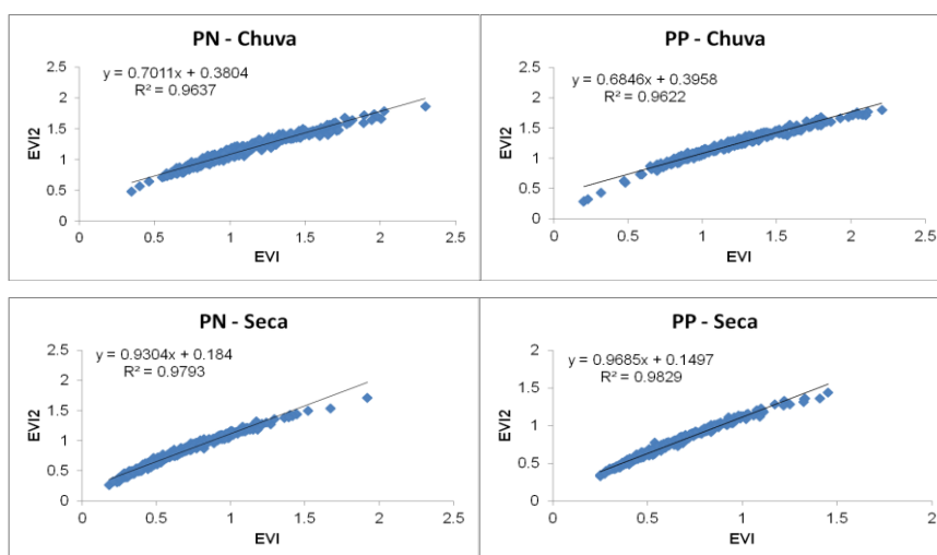
Figura 2. Gráficos de correlação entre os IVs para PP e PN em diferentes períodos sazonais.
