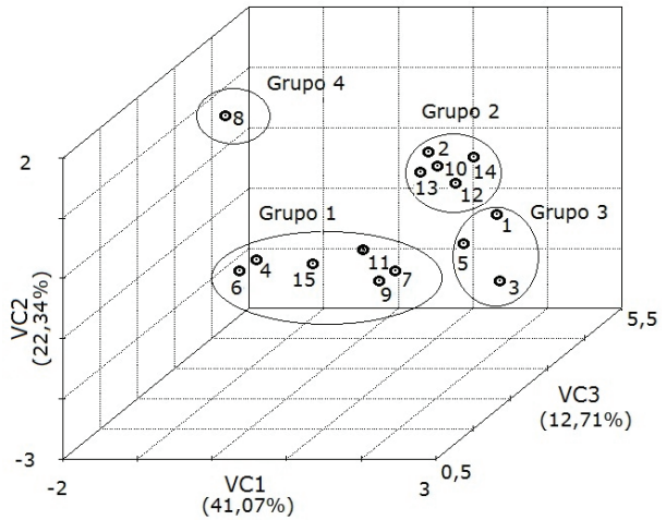
Figura 2. Dispersão gráfica dos escores dos caracteres morfoagronômicos, em relação aos três eixos principais de variáveis canônicas (VC1, VC2 e VC3), avaliados em quinze populações de pimenta longa (Rio Branco, AC, 2012).
