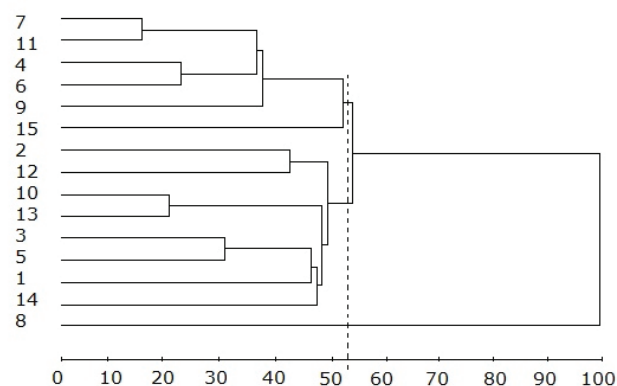
Figura 1. Dendrograma de dissimilaridades genéticas entre quinze populações de pimenta longa, obtido pelo método do vizinho mais próximo, com base nas distâncias generalizadas de Mahalanobis, para oito caracteres morfoagronômicos (corte, na distância, igual a 53%) (Rio Branco, AC, 2012).
