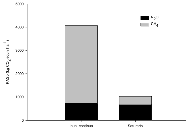
Figura 2. Potencial de aquecimento global em cultivo de arroz irrigado, sob distintos manejos da água.
