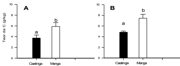
Figura 2. Teores de carbono na fração humina (A) e carbono orgânico total (B) em área com caatinga e com manga na cidade de Petrolina-PE.
