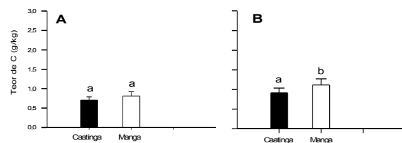
Figura 1. Teores de carbono das frações ácido fúlvico (A) e ácido húmico (B) em área com manga irrigada e caatinga nativa no município de Petrolina-PE.
