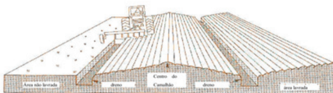
Figura 2.1 Confeção de camalhões de base larga.
