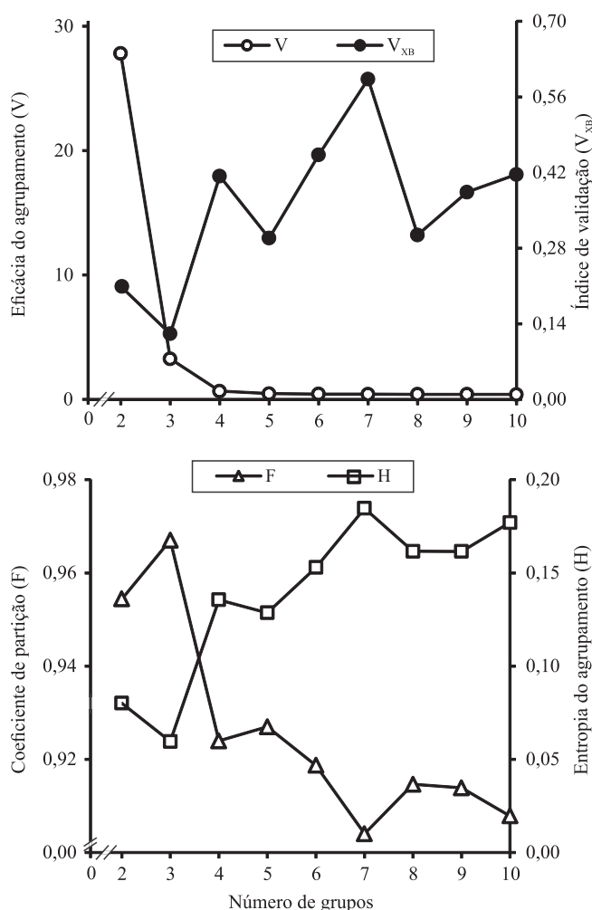
Figura 3. Parâmetros de avaliação dos agrupamentos obtidos pelo algoritmo "fuzzy c-means".
