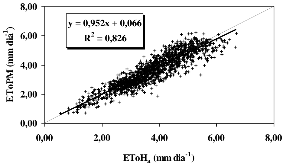
FIGURA 2 - Regressão linear entre os valores diários da evapotranspiração de referência estimados pelos métodos de Hargreaves ajustado (ETToHa) e o de Penman-Monteith (ETToPM). Jales, SP, 2005-2011 (anos ímpares).
