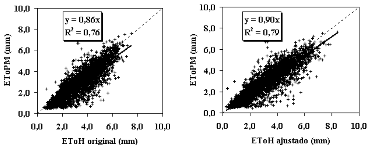
Figura 1 – Relação entre valores da evapotranspiração de referência estimada pelo método de Hargreaves (ET oH ) original e ajustado, em relação ao método padrão de Penman-Monteith (ET oPM ), para Bento Gonçalves, RS.
