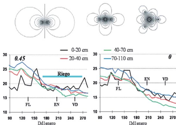
Figura 10. Evolución estacional del contenido de humedad del suelo (%v/v), medido con TDR, a distintas profundidades para los tratamientos de riego con k_c = 0.45 (izquierda) y seco k_c = 0.0 (derecha)
